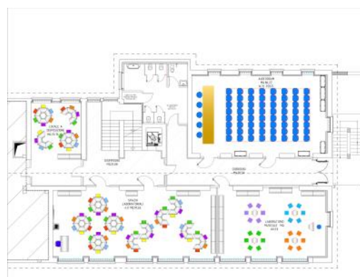
Planimetria di progetto del sottotetto
